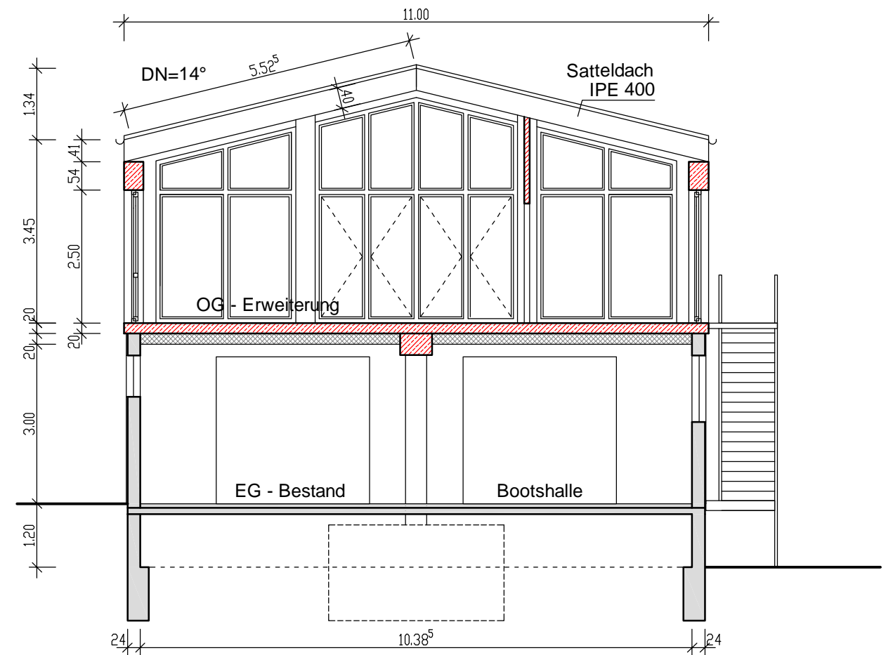
Schnitt B-B
