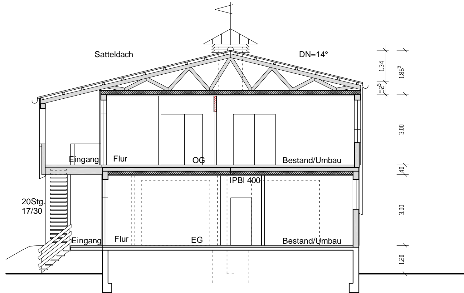
Schnitt A-A Bestand
